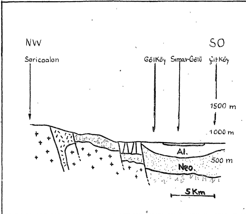
Schnitt A, Profilskizze des Simav-Grabens, vergleiche Abb. 2
