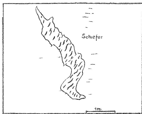
Abb. 4 «Pegmatit», westlich Demirci-Koy (Sinav)? schwarz = Quarz, ausgewalzt, Rest Orthoklas
