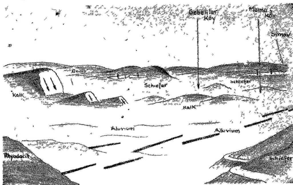
Abb 2 Blick von der Strasse Simav - Gediz in Richtung Südwesten. Links und im Hintergrund Treppenverwerfungen (Pfeilrichtung/)
