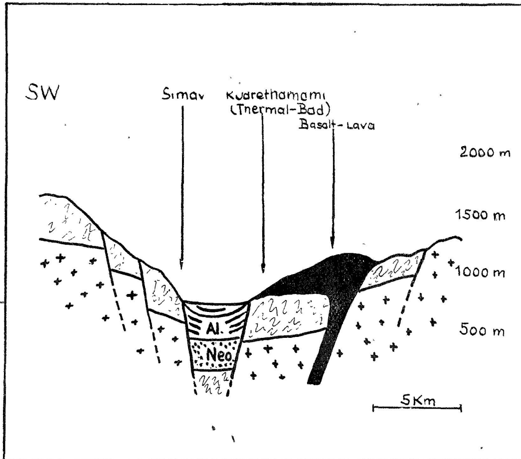
Schnitt B, Profilskizze des Simav - Grabens, vergleiche Abb. 2
