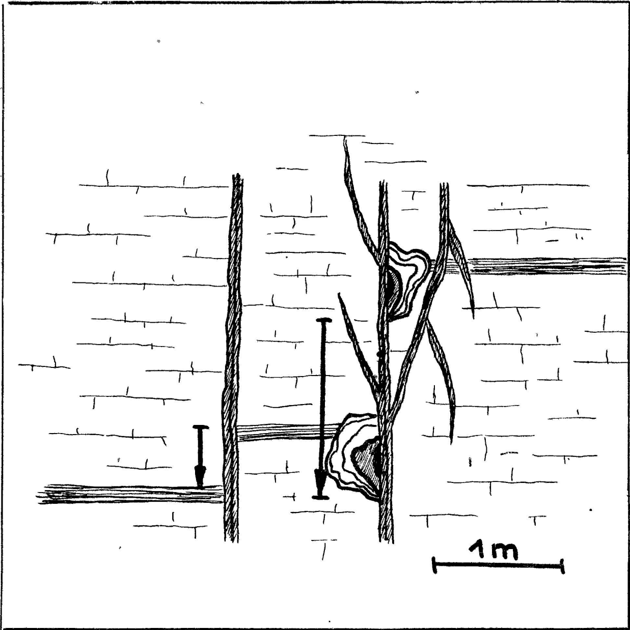
Abb. 3 Kleintektonik in einem Kalksteinbruch oberhalb der Stadt Siinav. Pfeile deuten Verwerfungsrichtungen an. Risse sind mit Aragonit ausgeheilt.
